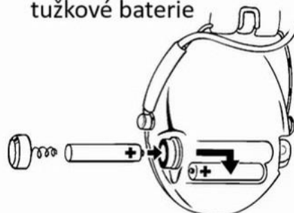
Směr a pozice tužkové baterie
